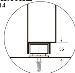
SIMPLE / DOUBLE Détail 4
