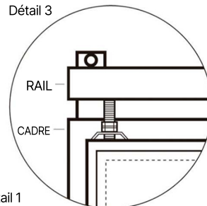
SIMPLE Détail 3
